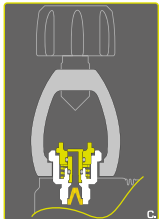
Figure C : Détendeur non connecté en étrier > détendeur obstrué
