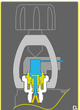
Figure D : Détendeur non connecté en étrier > détendeur ouvert
